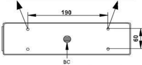
Soket Yerleri-Place Of Socket-Anschluss-Place Du Socle
