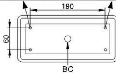
Soket Yerleri-Place Of Socket-Anschluss-Place Du Socle
