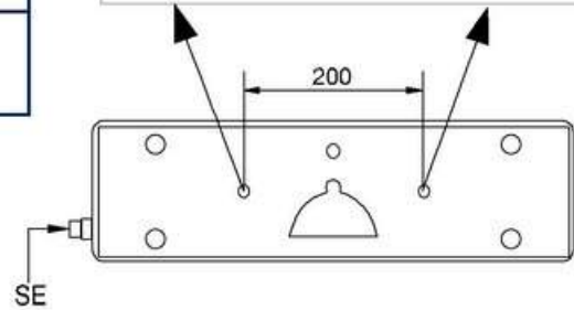
Soket Yerleri-Place Of Socket-Anschluss-Place Du Socle
