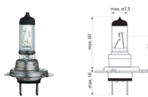
H7 - Px 26d
